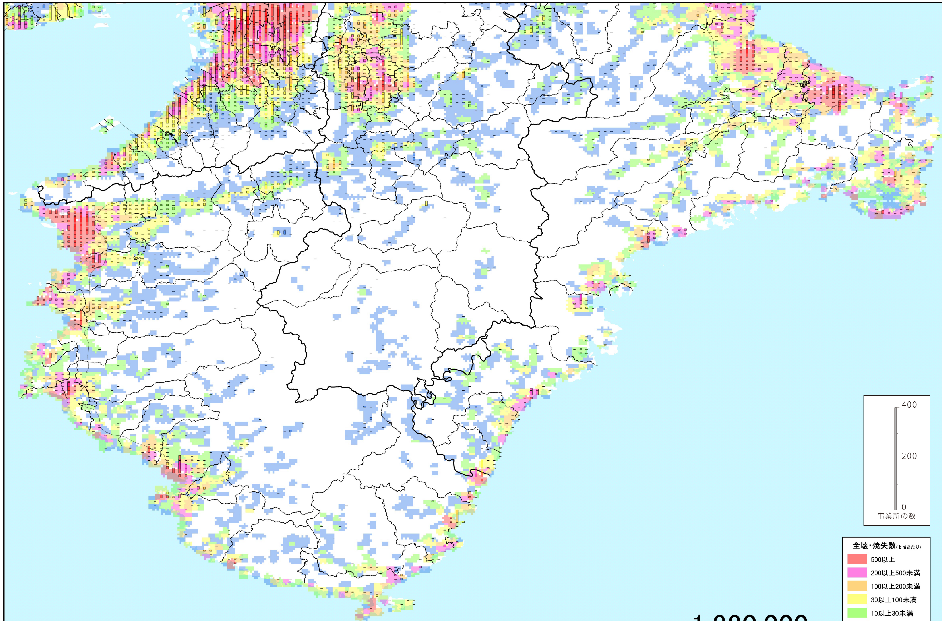
南海トラフ巨大地震 全壊・焼失数×食品小売業事業所数[紀伊半島]
