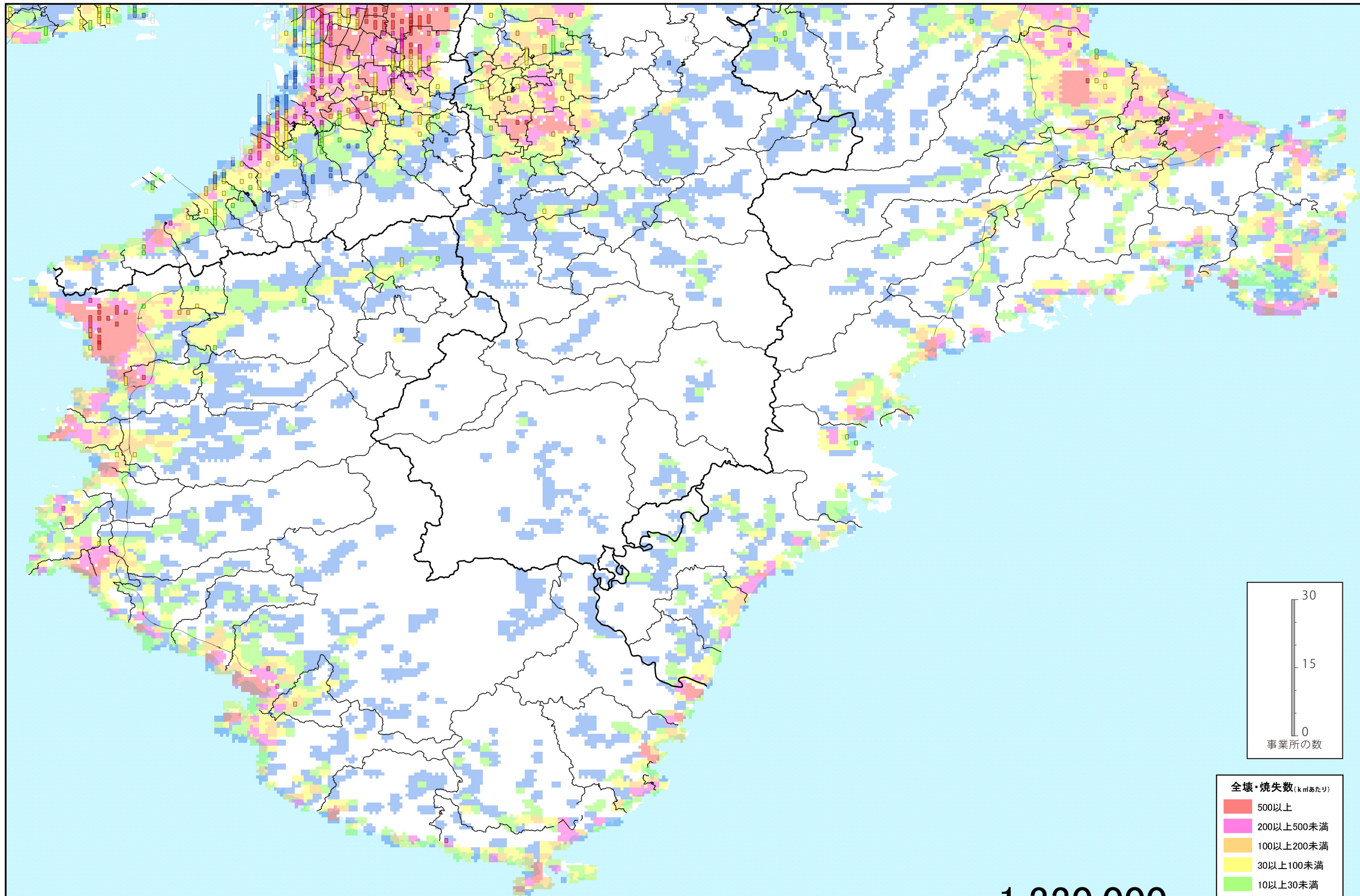
南海トラフ巨大地震 全壊・焼失数×倉庫業事業所数[紀伊半島]
